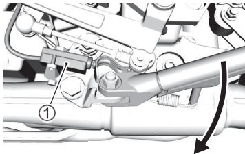
1. Interruptor do descanso lateral / intertravamento de ignição
